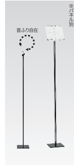
S-61 サインスタンド W200・D200・H1200 本体:ブラック、スチール パネル取付面:W100・H100 ※パネル取り付け方法: ホネジ又は両面テープ 首振り自在
