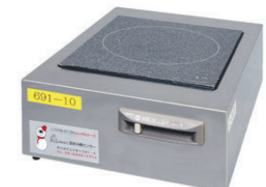
電磁調理器 単相200V 2.0KW K69-1 外形寸法 W300×D453×H100mm 電 源 単相200V2.0KW
