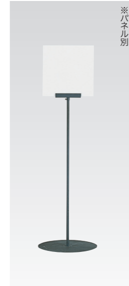
S-64 サインスタンド φ350・H900~1200 ホルダー部:W150・H20 スウェードグレー塗装 スライドインクリップ式 対応パネル:厚さ5mmまで
