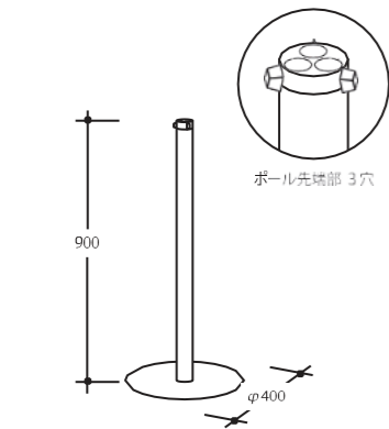
MUP ユニットポール本体 H900
